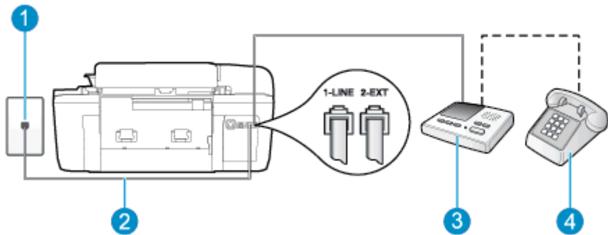
图 B-12 打印机的后视图
